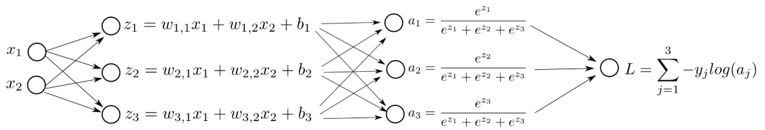
Figura 4.2: Flusso della regressione softmax con due ingressi e tre classi: dai logit z_i = w_{i,1}x_1 + w_{i,2}x_2 + b_i alle probabilità a_i = \frac{e^{z_i}}{\sum_{k=1}^3 e^{z_k}} , fino alla loss a entropia incrociata L = \sum_{j=1}^3 -y_j \log(a_j) .
