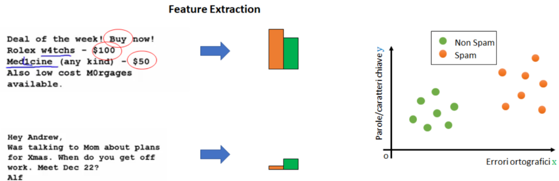
Figura 1.1: Estrazione delle feature: le e-mail vengono trasformate in vettori 2D, dove x = errori ortografici e y = pattern ripetibili, e proiettate nello spazio delle feature, , dove la separazione tra spam (arancione) e non spam (verde) risulta evidente.
