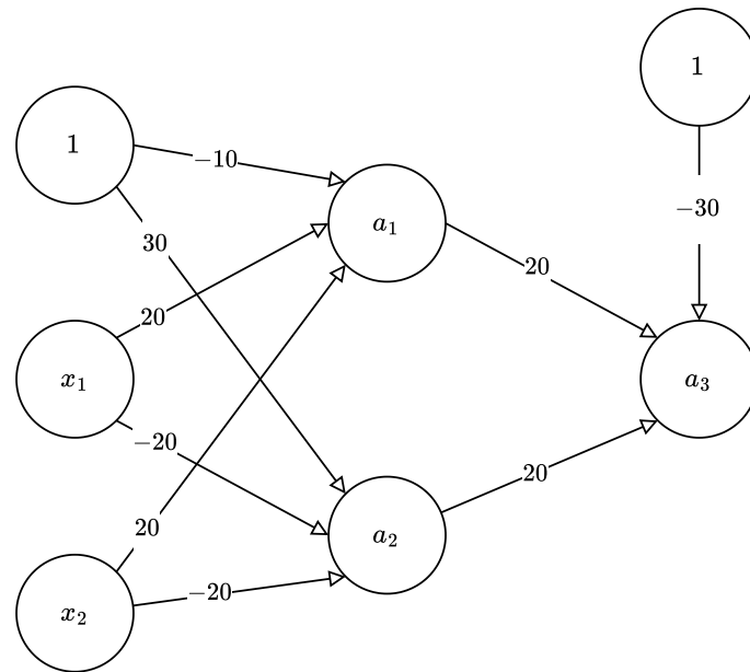
Figura 2.5: Rete di percettroni per computare lo XOR
