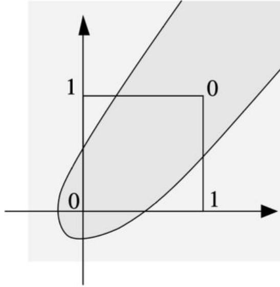
Figura 2.4: Schema del problema XOR: i vertici (0,1) e (1,0) appartengono alla classe 1, (0,0) e (1,1) alla classe 0. Nessuna frontiera lineare può separare le classi; è necessaria una frontiera non lineare (ottenibile con uno strato nascosto).
