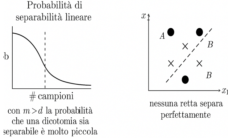
Figura A.1: Separabilità non lineare. A sinistra: andamento qualitativo della probabilità che una dicotomia sia linearmente separabile al crescere del numero di campioni m (con dimensione d fissata); a destra: esempio in \mathbb{R}^2 di punti non separabili con un singolo iperpiano.
